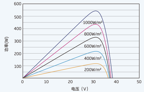
组件的P-V曲线 (545W)
