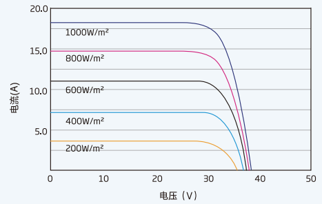
组件的I-V曲线 (545W)
